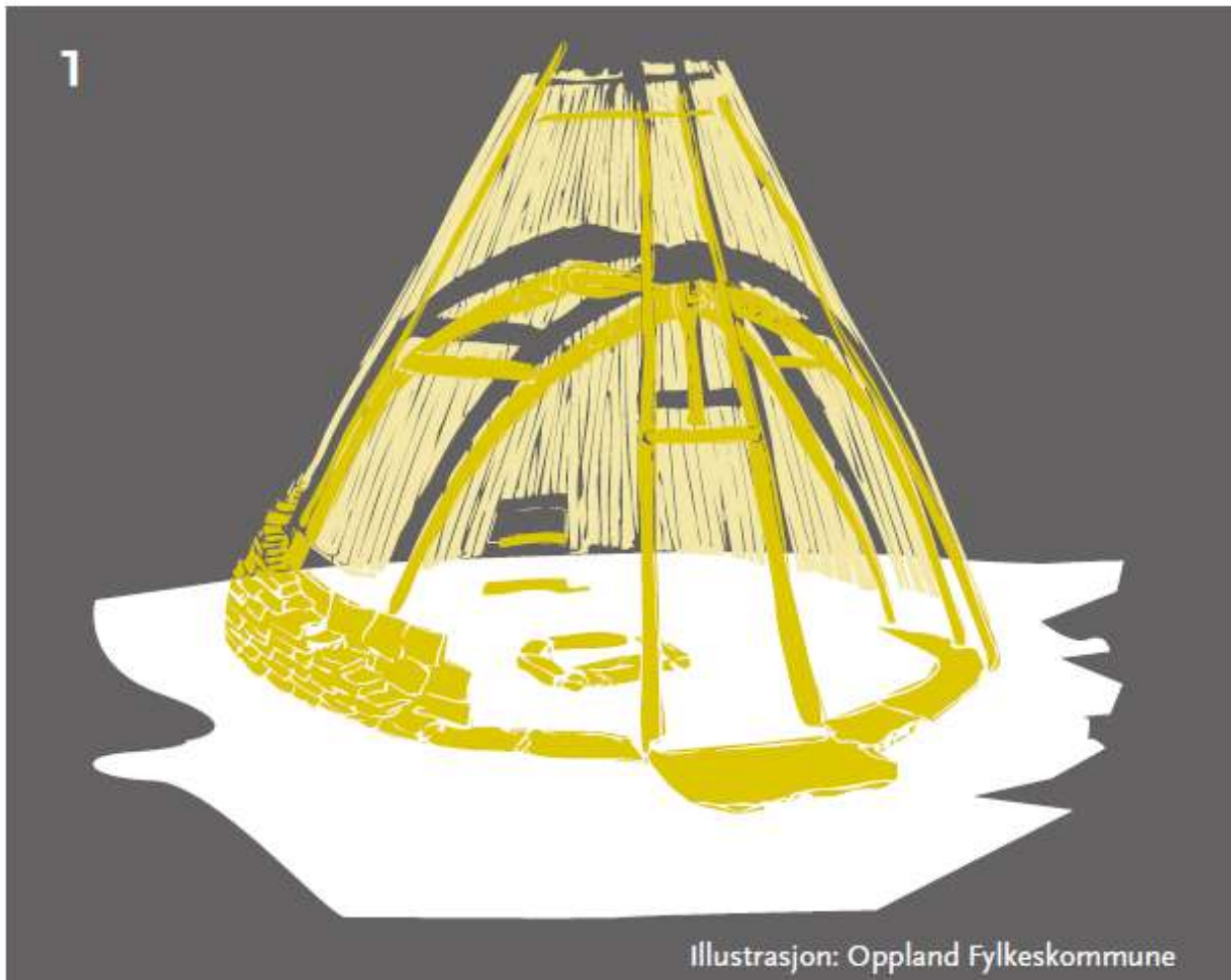
Figur 84. Teikning av sametufta slik ho kan sjå ut. Kjelde: Oppland fylkeskommune
