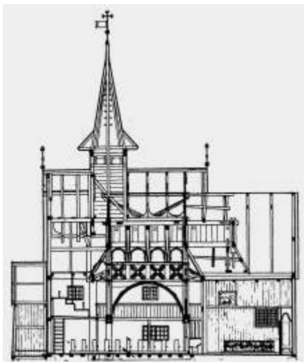
Figur 39. Kyrjekonstruksjonen. Berre den midtre delen med boge, overbygg og framparti mot høgre er den opphavlege stavkyrkja.
